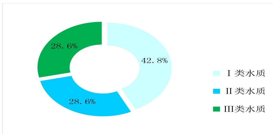
图 1 安顺市县级以上集中式饮用水水质达标类别状况
