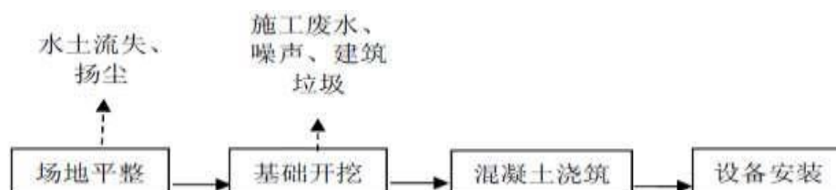
图 2-3 箱式变压器及逆变器施工共计及产污环节
