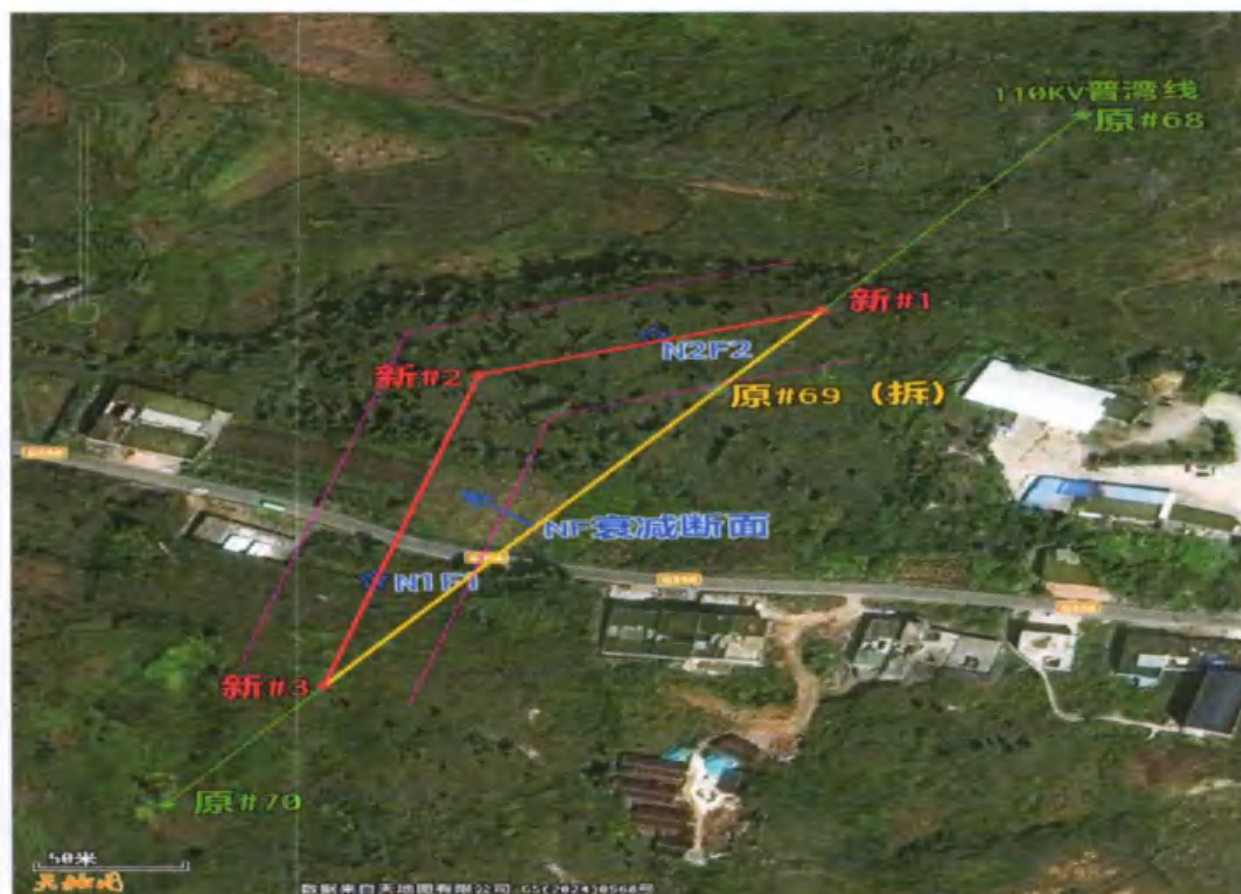
110 千伏普湾线监测布点示意图
