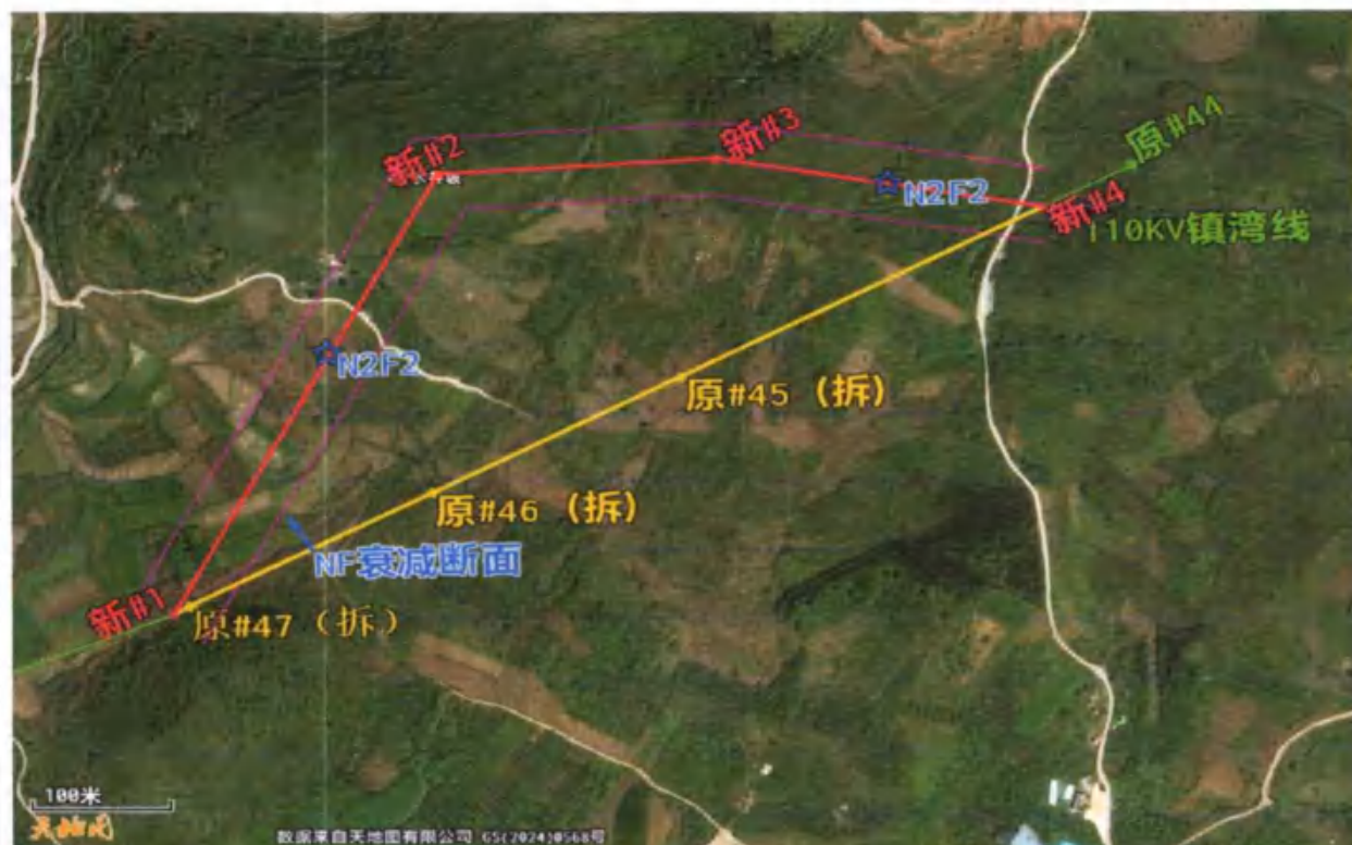
110 千伏镇湾线监测布点示意图
